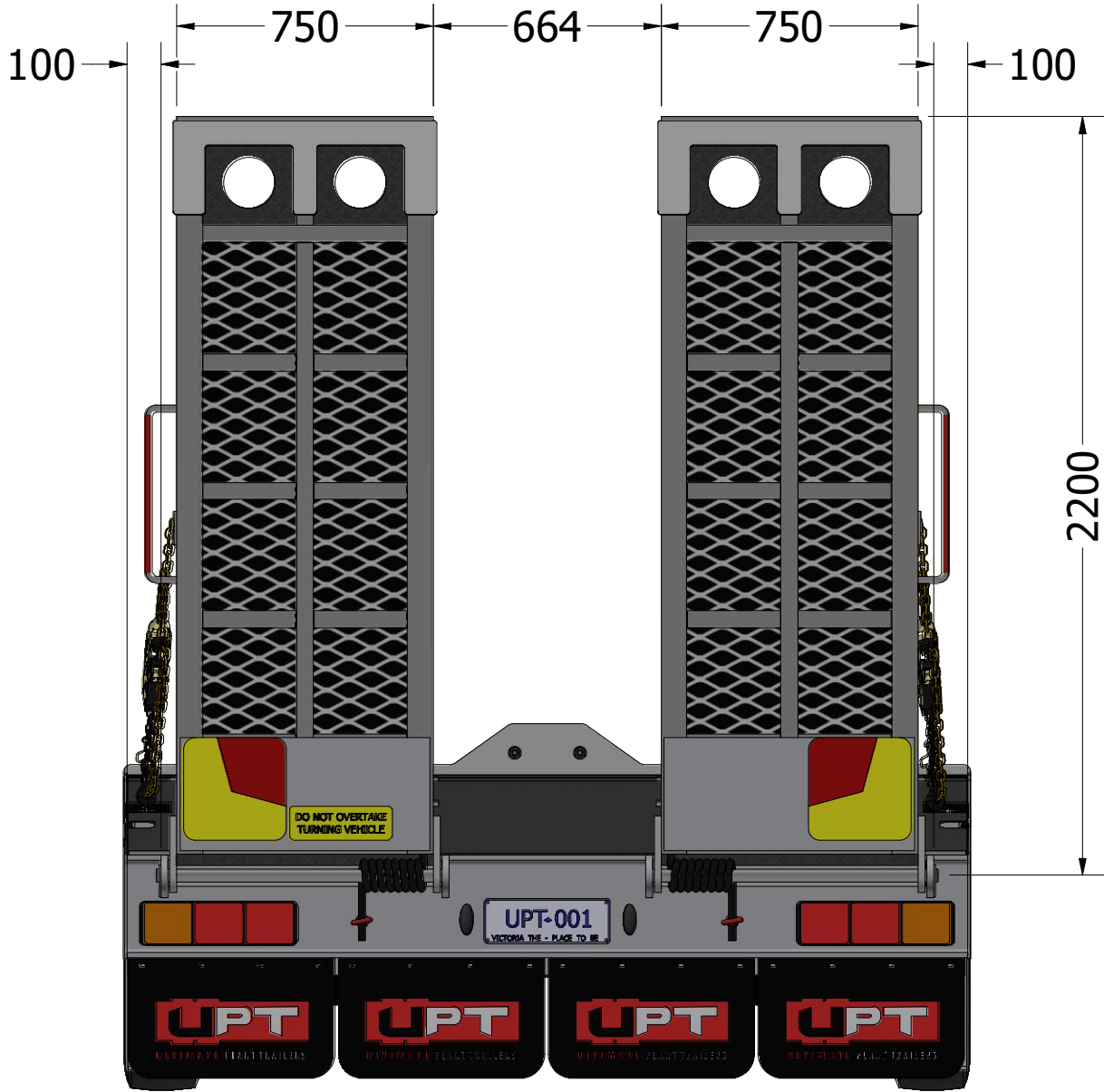
9T TANDEM
